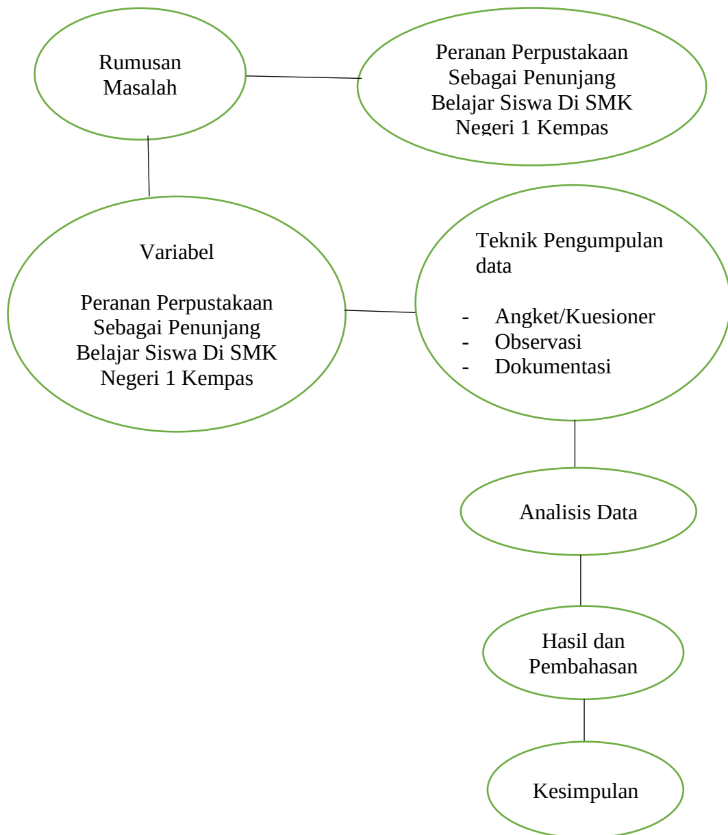
Gambar 1. Desain Penelitian
