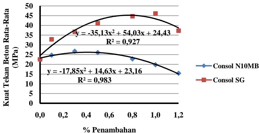
Gambar 1. Hubungan Persentase Penambahan Consol N10MB dan Consol SG terhadap Kuat Tekan Beton
