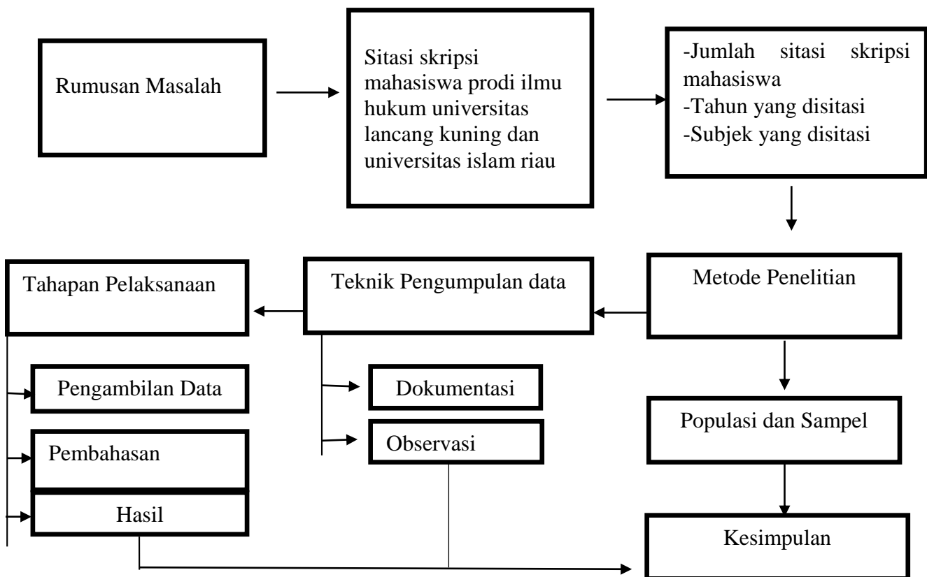
Gambar 1. Desain Penelitian
